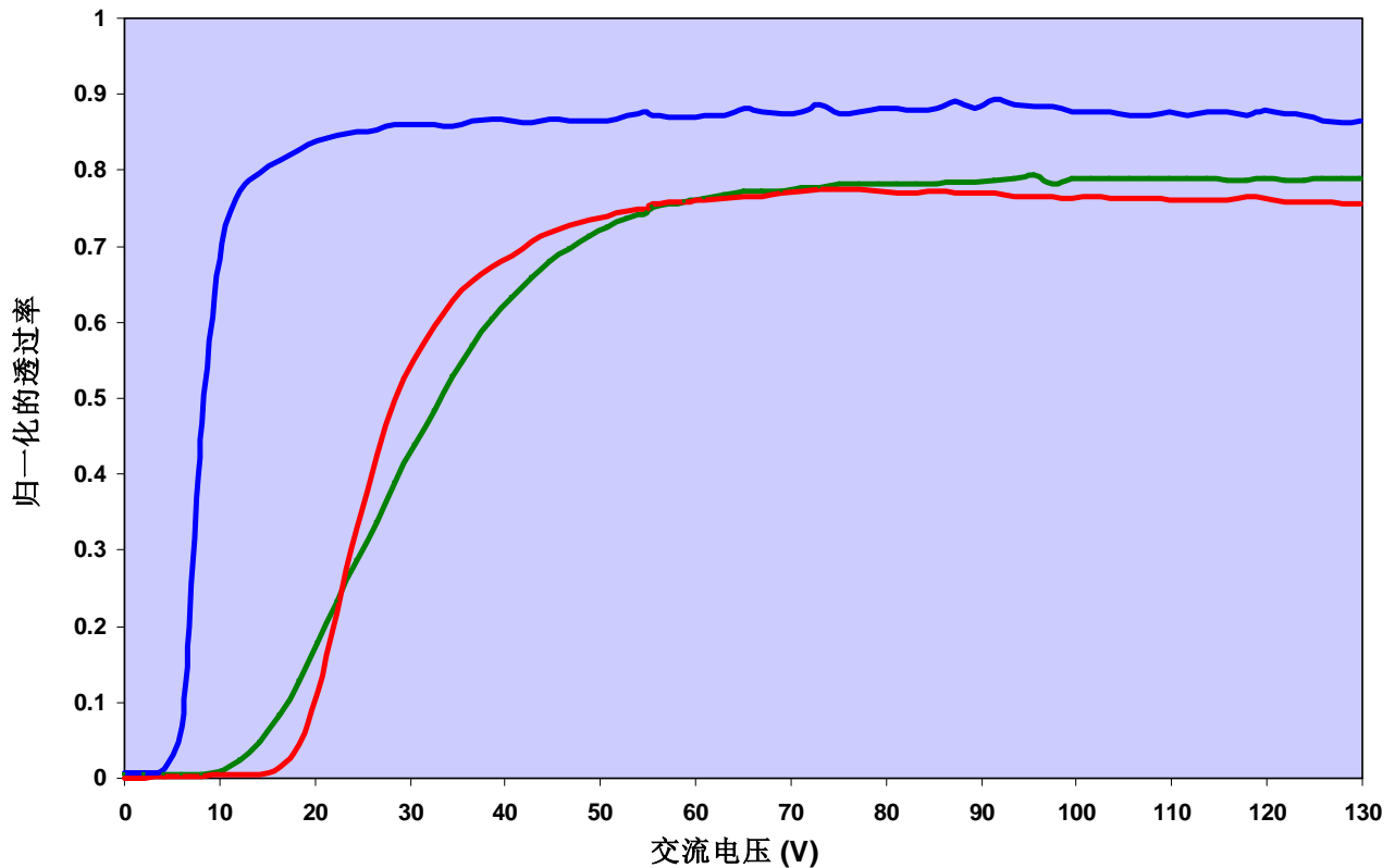
不同代的液晶微粒显示器的光电曲线比较
