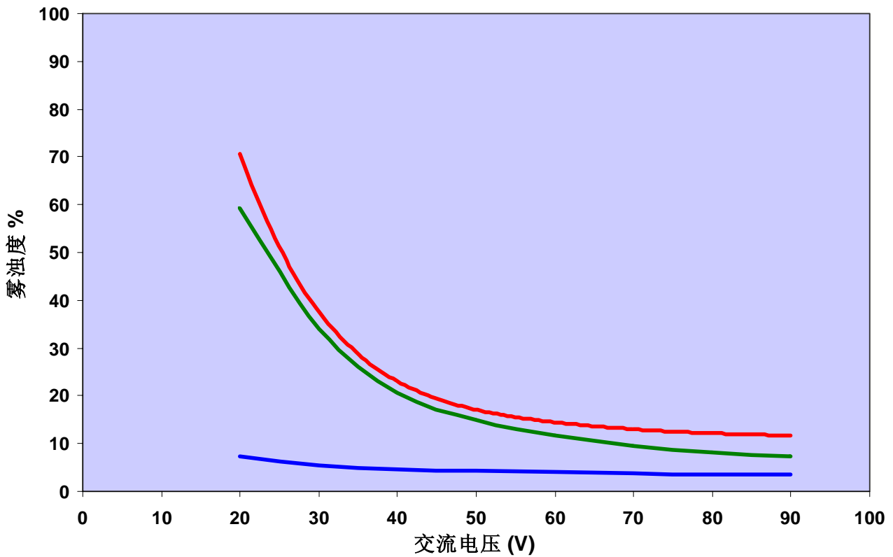
不同代的液晶微粒显示器的雾浊度-电压曲线的比较
